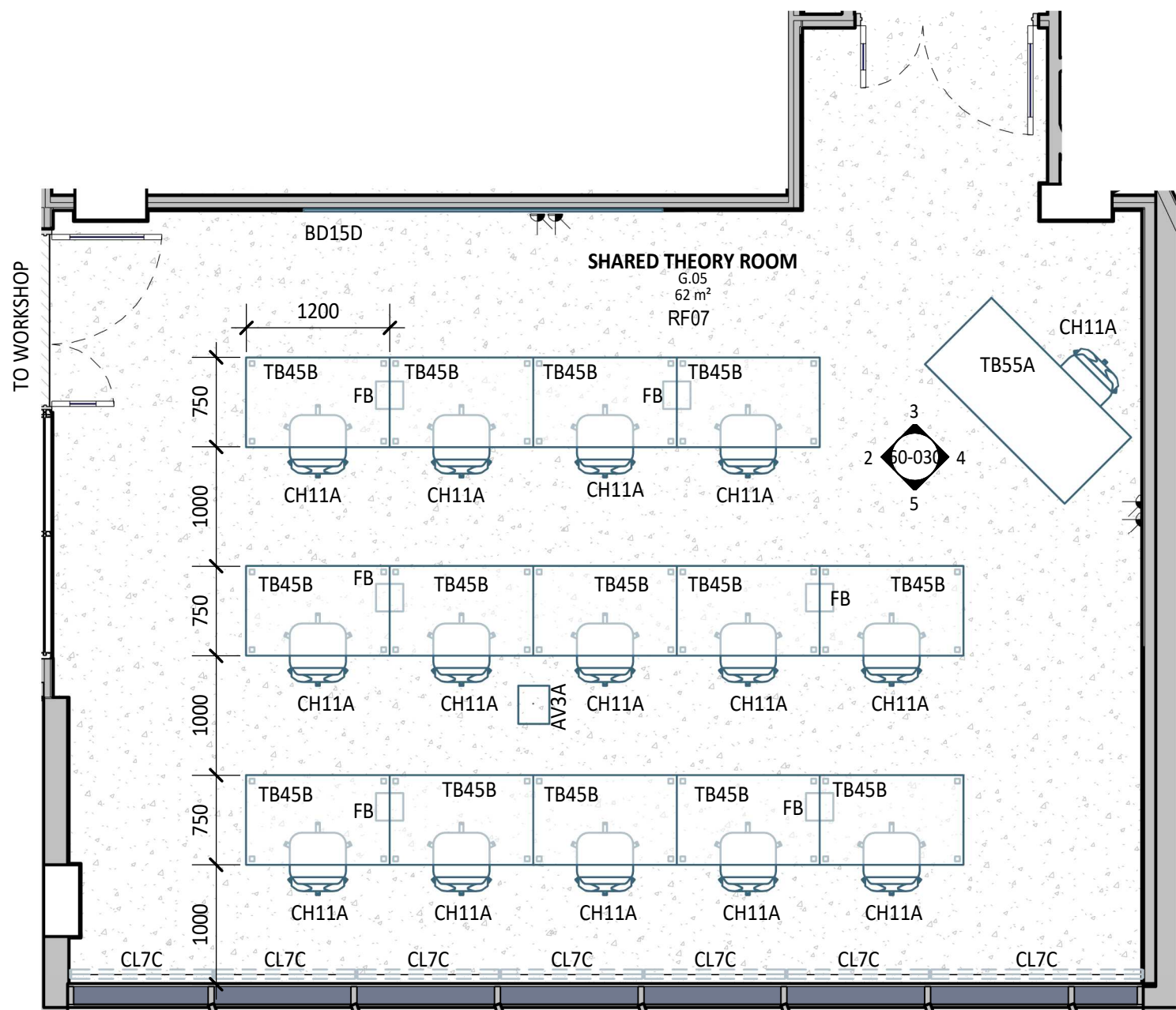
1 PLAN DETAIL 1 : 50
